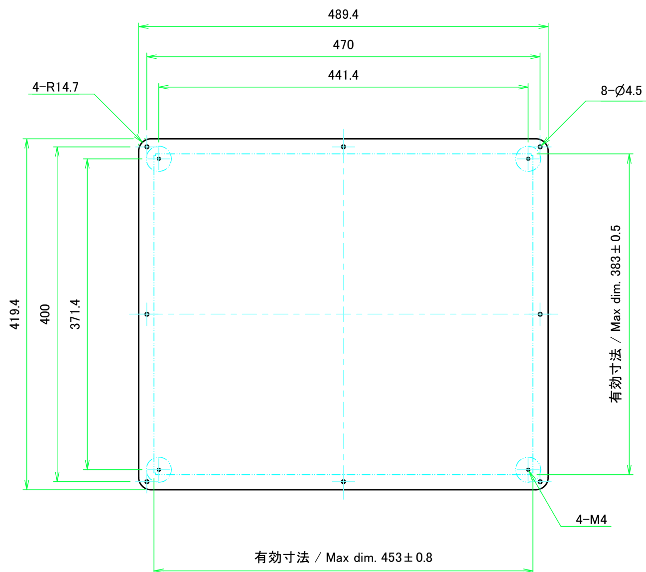
保護シート側 Surface protective film side
