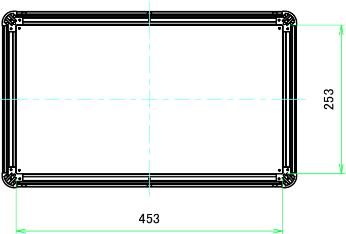
B-B ( 1:6.5 )
