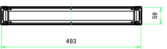
C-C ( 1:6.5 )
