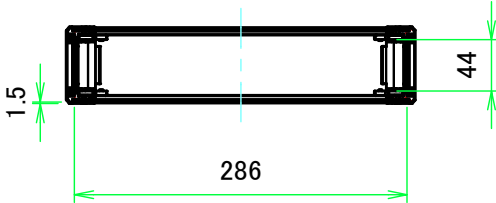
A-A ( 1:6.5 )
