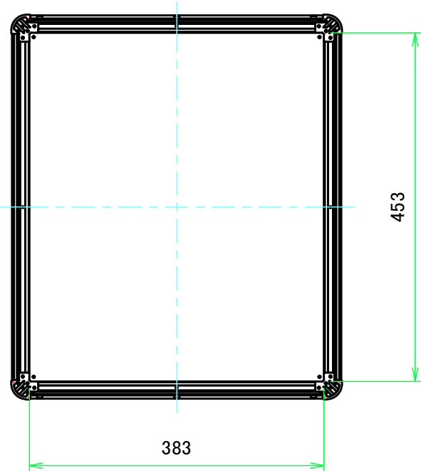
B-B ( 1:7 )
