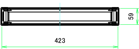
C-C ( 1:7 )
