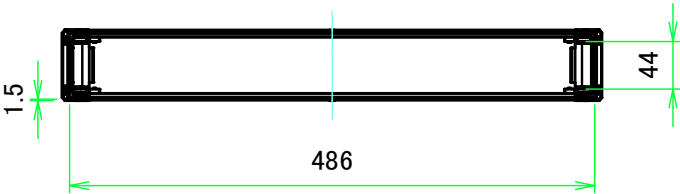
A-A ( 1:7 )
