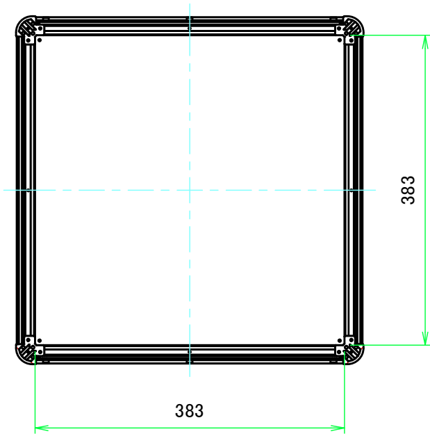
B-B ( 1:6.5 )
