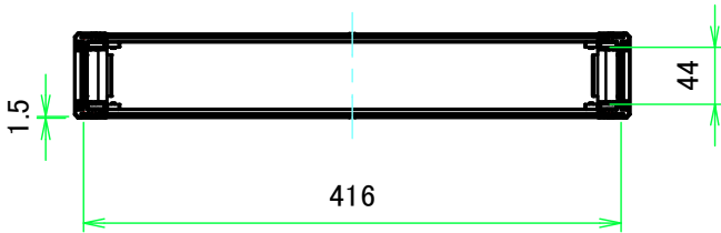
A-A ( 1:6.5 )
