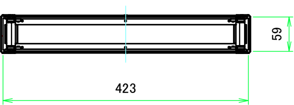
C-C ( 1:6.5 )
