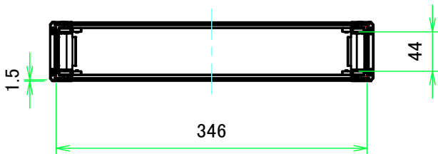
A-A ( 1:6 )
