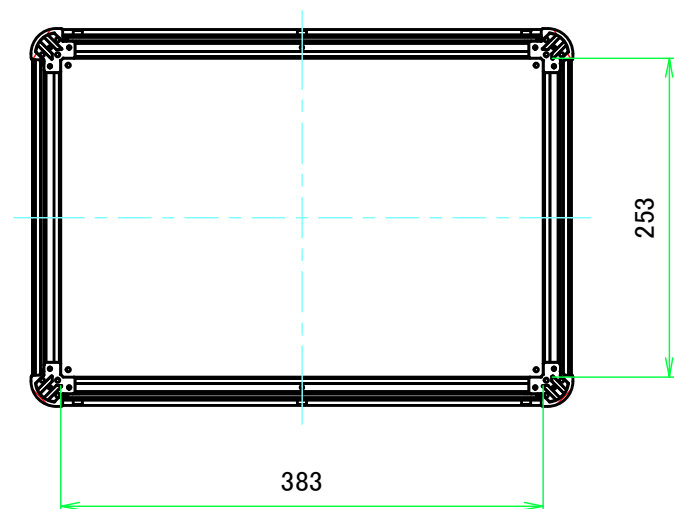
B-B ( 1:6 )
