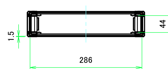
A-A ( 1:6 )
