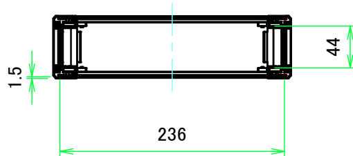
A-A ( 1:5.5 )
