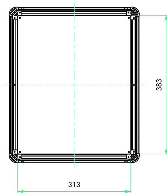
B-B ( 1:6 )
