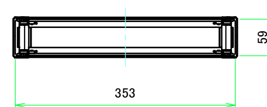
C-C ( 1:6 )
