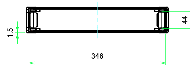
A-A ( 1:5.5 )
