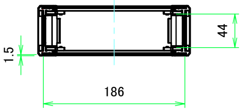
A-A ( 1:5 )
