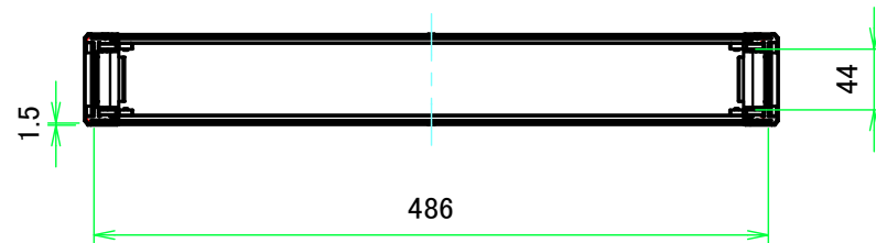
A-A ( 1:6 )
