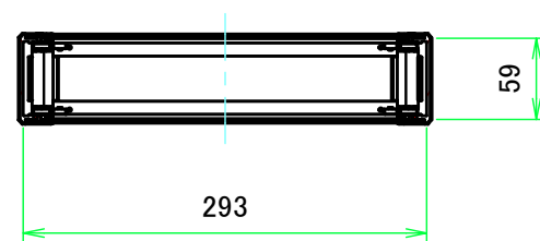
C-C ( 1:6 )
