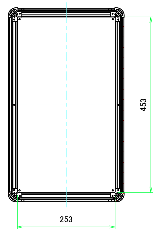
B-B ( 1:6 )
