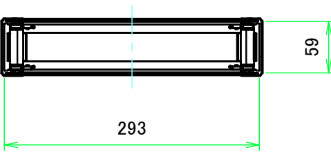
C-C ( 1:6 )
