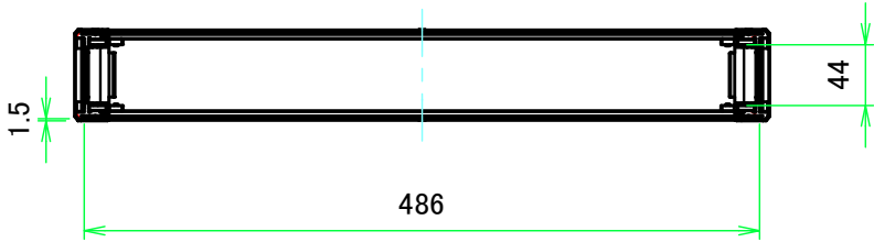
A-A ( 1:6 )
