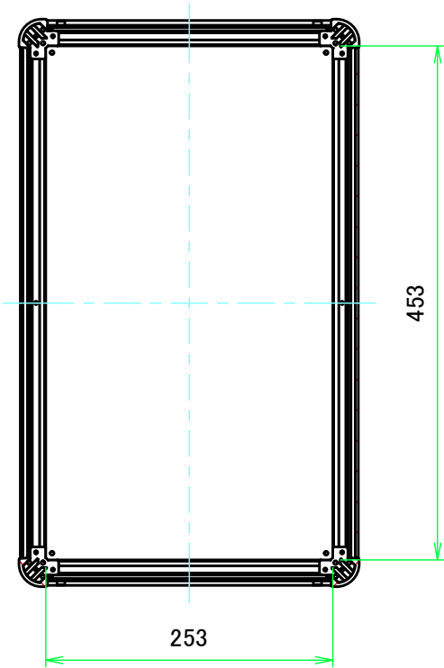
B-B ( 1:6 )
