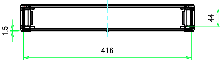
A-A ( 1:5.5 )
