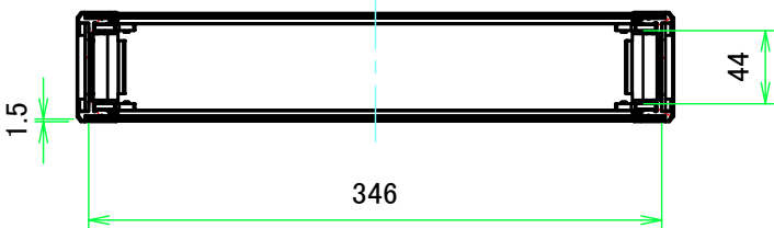
A-A ( 1:5 )
