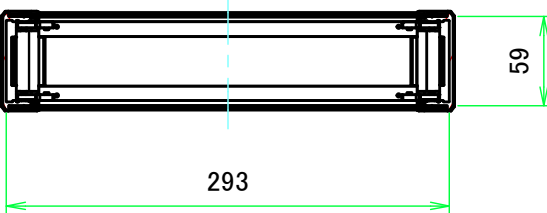
C-C ( 1:5 )
