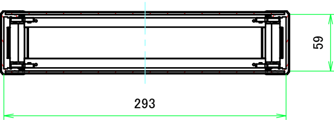
C-C ( 1:4 )
