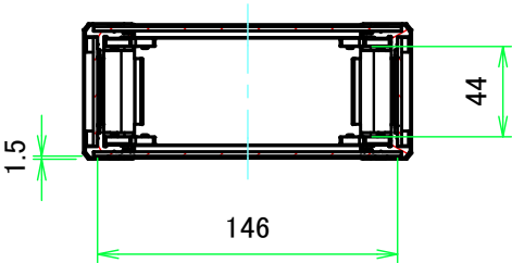
A-A ( 1:4 )
