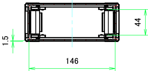
A-A ( 1:4 )
