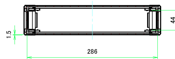
A-A ( 1:4 )
