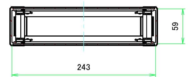
C-C ( 1:4 )
