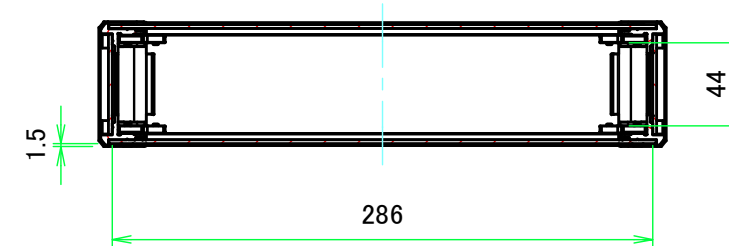
A-A ( 1:4 )
