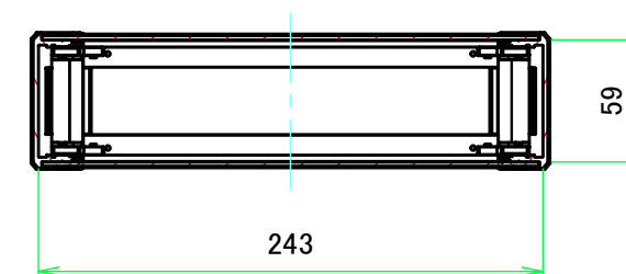
C-C ( 1:4 )
