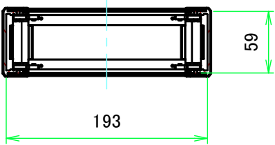
C-C ( 1:5 )
