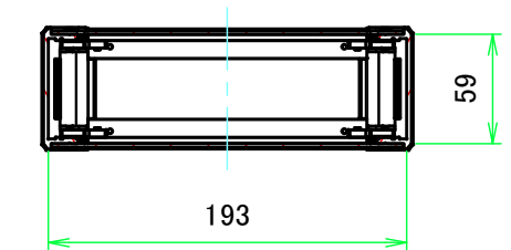
C-C ( 1:4.5 )
