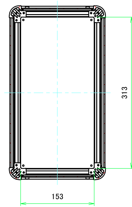
B-B ( 1:4.5 )
