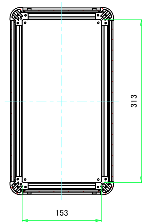
B-B ( 1:4.5 )
