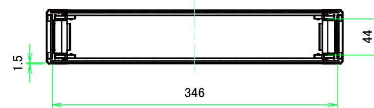
A-A ( 1:4.5 )
