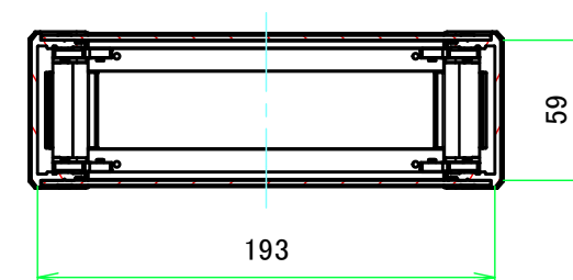
C-C ( 1:3.5 )
