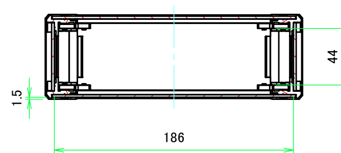
A-A ( 1:3 )
