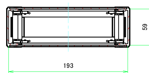
C-C ( 1:3 )
