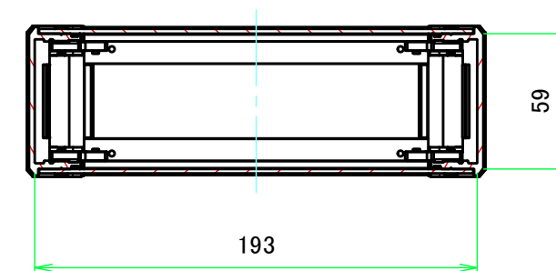
C-C ( 1:3 )
