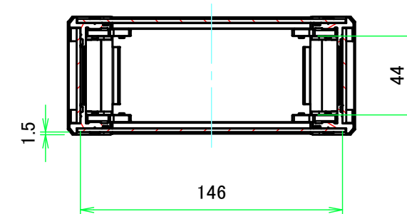
A-A ( 1:3 )
