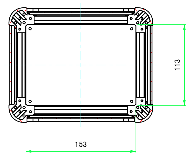
B-B ( 1:3 )
