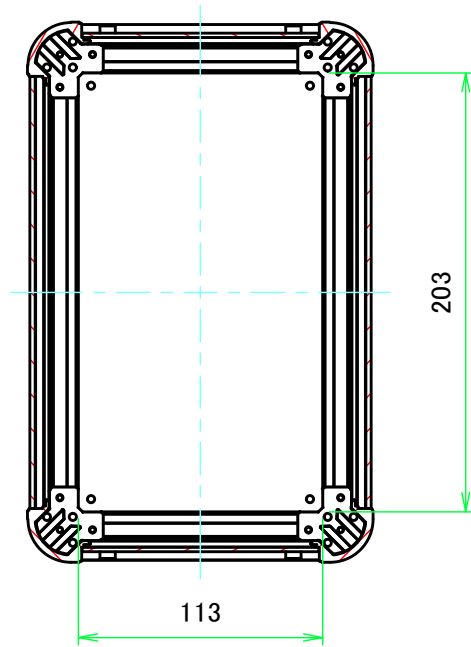
B-B ( 1:3.5 )
