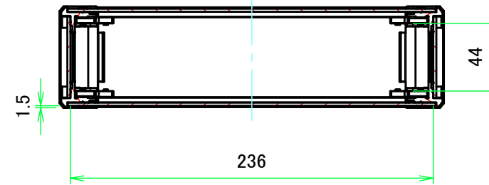
A-A ( 1:3.5 )
