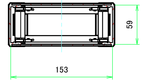
C-C ( 1:3.5 )
