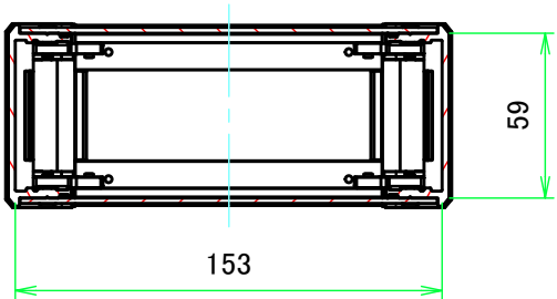
C-C ( 1:3 )
