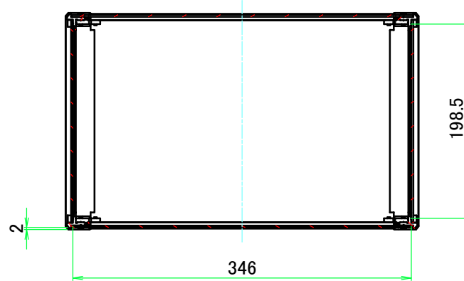
A-A ( 1 : 5.5 )
