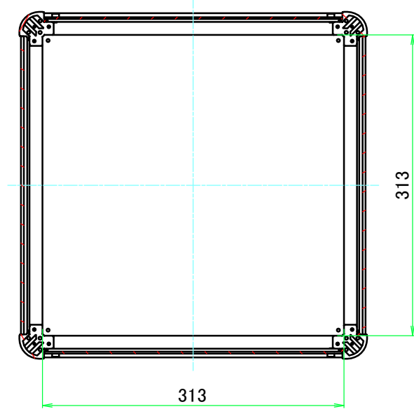
B-B ( 1 : 5.5 )
