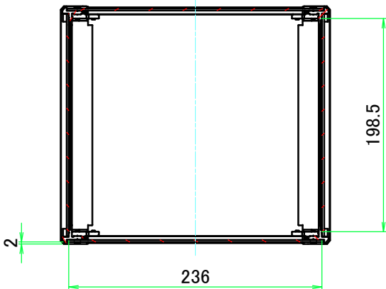
A-A ( 1 : 5 )
