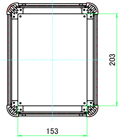
B-B ( 1 : 5 )
