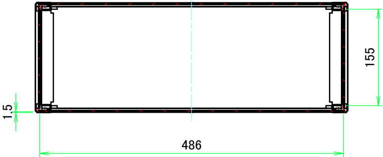
A-A ( 1 : 6 )
