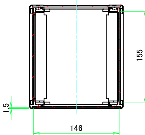
A-A ( 1 : 4 )
