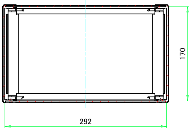
C-C ( 1 : 4 )
