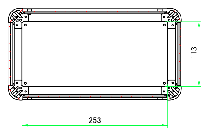
B-B ( 1 : 4 )
