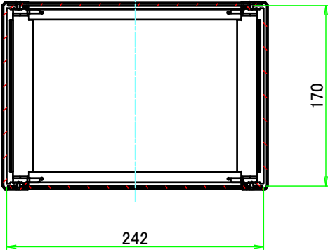
C-C ( 1 : 5 )
