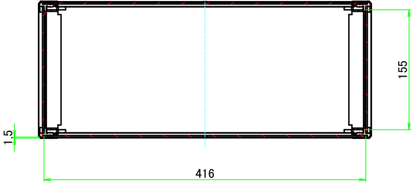
A-A ( 1 : 5 )
