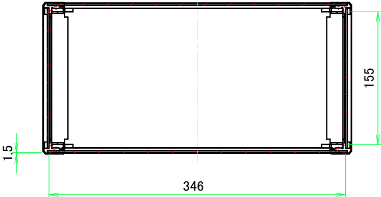
A-A ( 1 :4.5 )
