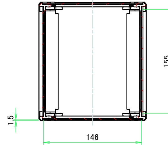
A-A ( 1 :3.5 )
