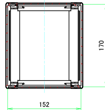
C-C ( 1 : 4 )
