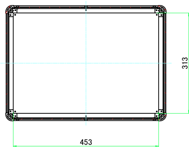
B-B ( 1 : 7 )
