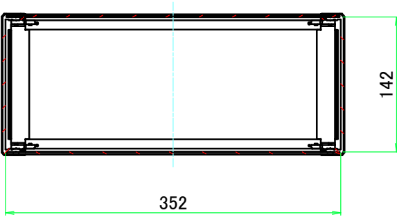
C-C ( 1 : 5.5 )
