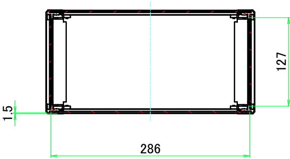
A-A ( 1 : 5.5 )
