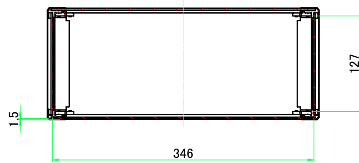
A-A (1:5)
