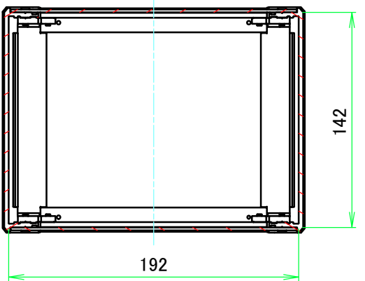
C-C ( 1 : 3.5 )
