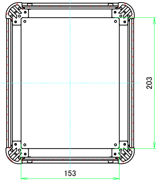
B-B ( 1 : 3.5 )
