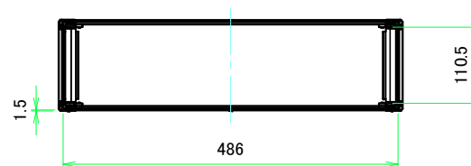
A-A (1:7)
