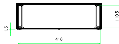
A-A (1:6.5)
