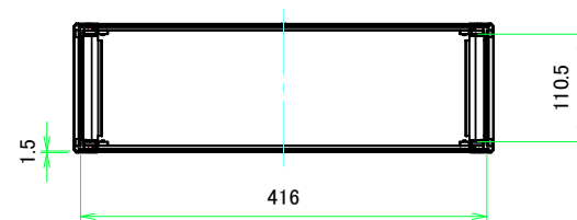
A-A (1:6)
