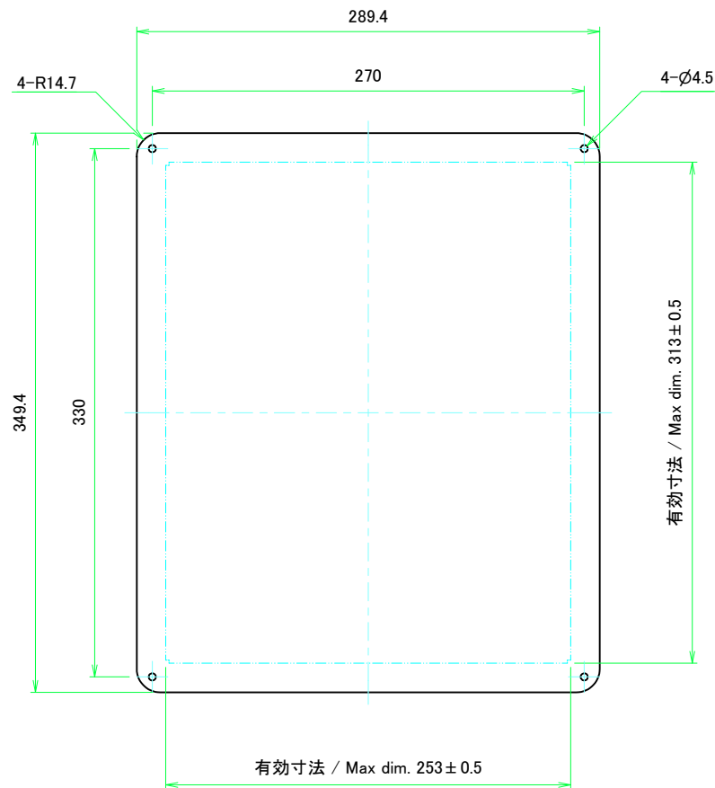
保護シート側 Surface protective film side
