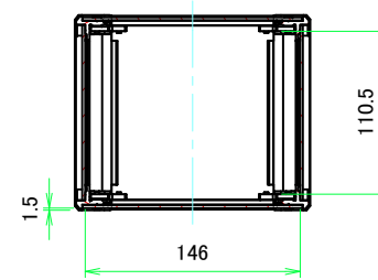
A-A (1:4)
