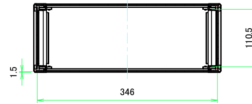
A-A (1:5)
