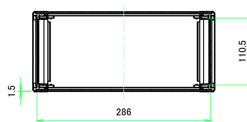
A-A (1:4.5)
