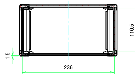
A-A (1:4)
