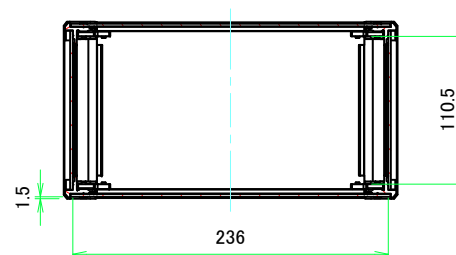
A-A (1:4)
